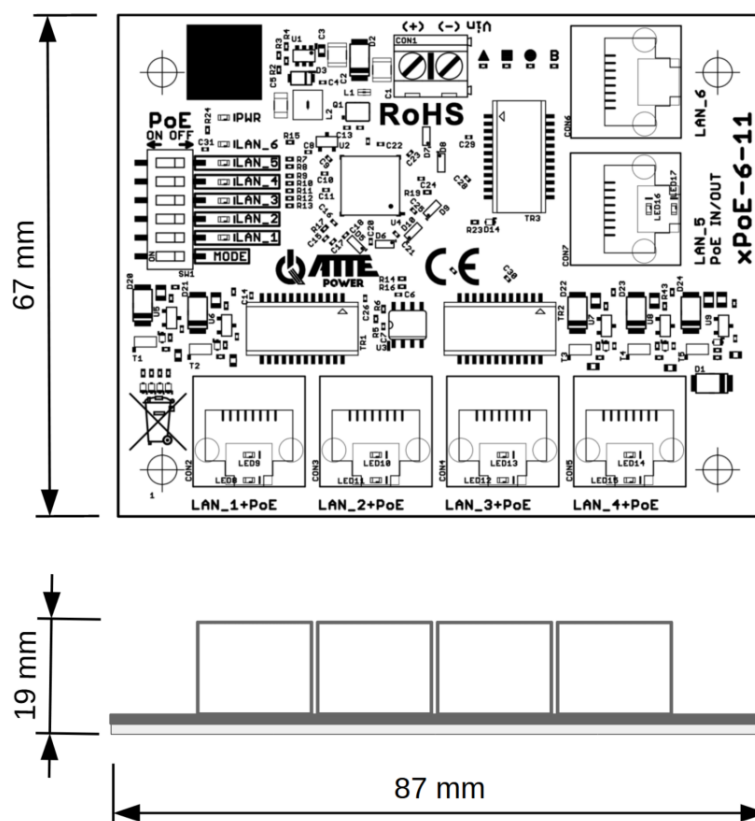
Ogólny widok urządzenia
